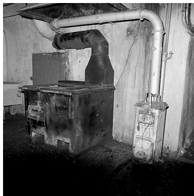
Cuisine et chaudière de chauffage central. Phot. Gérard Roucaute IVR93_19910400327X
